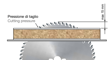
Con mordente positivo la pressione di taglio agisce sul piano di appoggio. With positive wood stain, the cutting pressure acts over the bearing plane.
