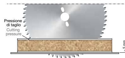
Con mordente negativo la pressione di taglio agisce sul piano di appoggio. With negative wood stain, the cutting pressure acts over the bearing plane.
